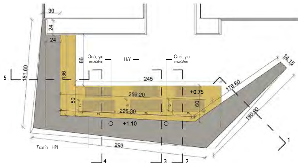
ΟΡΙΖΟΝΤΙΑ ΤΟΜΗ (+1,20)
