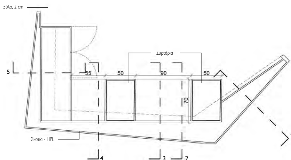
ΟΡΙΖΟΝΤΙΑ ΤΟΜΗ (+0,70)
